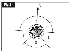
Figure 1 - Description de l'abattage : chemin de repli
