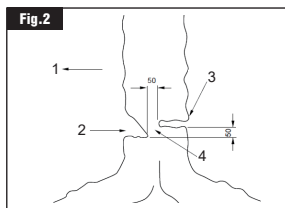
Figura 2 - Descrição do abate: corte a partir da base
