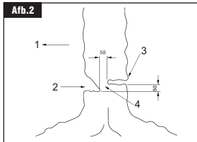
Afbeelding 2 - Beschrijving van het vellen: onderbokken
