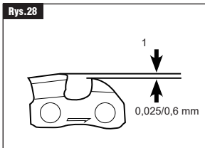
1. Przeświet głębokościomierza
