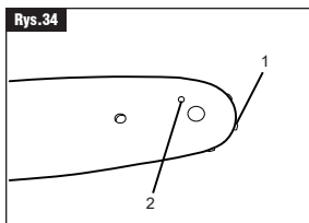
1. Koło łańcuchowe w końcówce prowadnicy 2. Otwór smarujący
